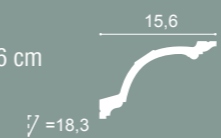
C217 | C217F 200 x 15,6 x 10,3 cm Purotouch®
