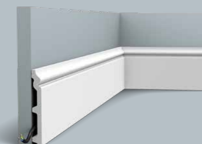
SX118 | SX118F | SX118-RAL9003 CONTOUR 200 x 13,9 x 1,8 cm Duropolymer®
