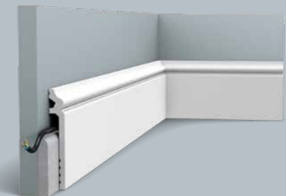
SX186 CONTOUR 200 x 13,8 x 2,2 cm Duopolymer ®
