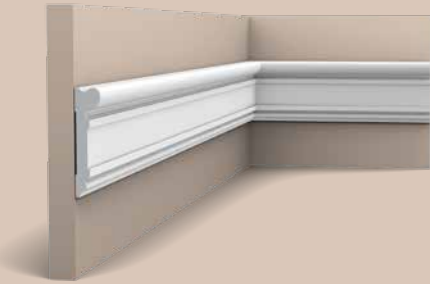
DX119-2300 230 x 9,2 x 2,2 cm Duropolymer®
